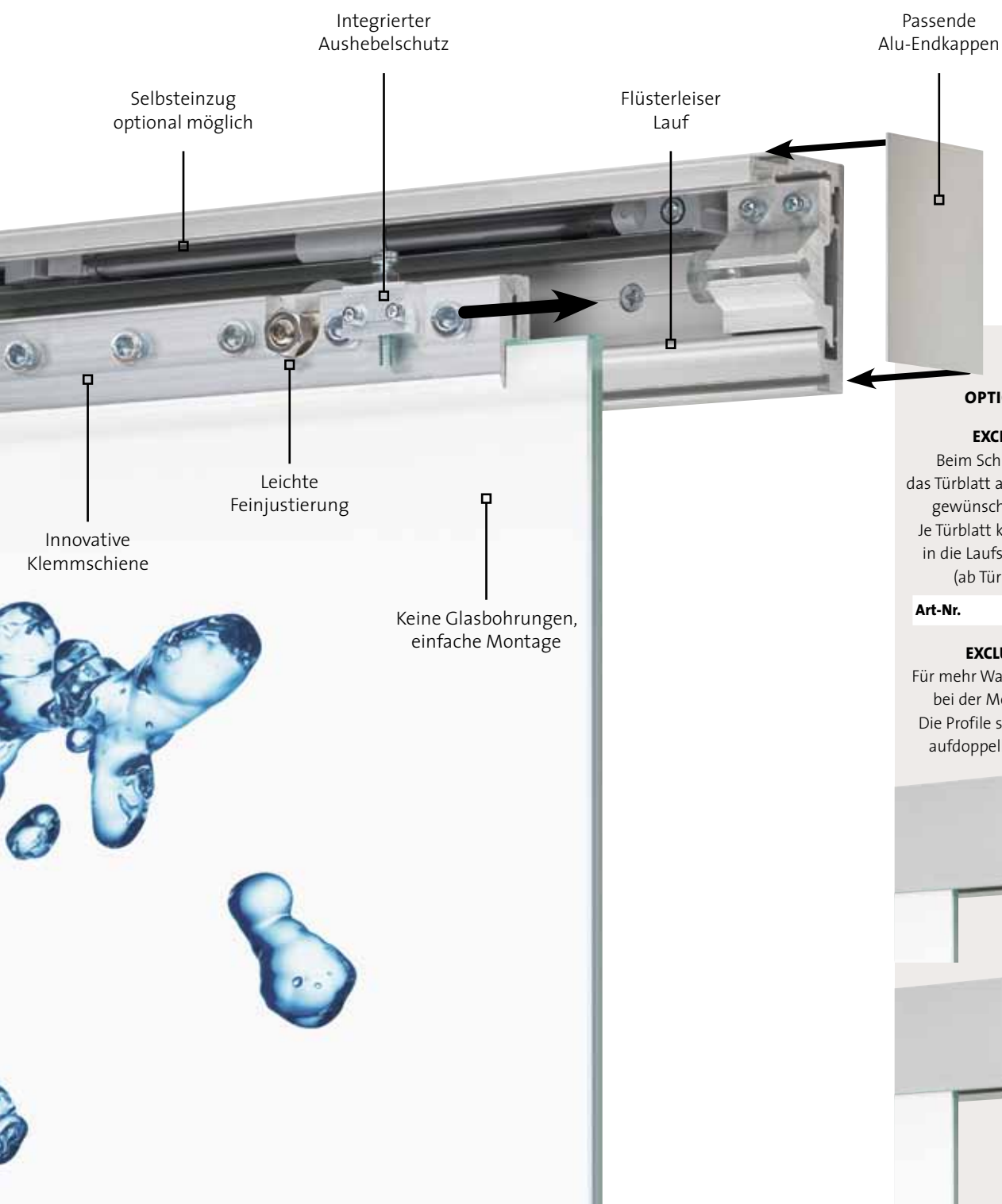
Einfache Unterfütterung Glas bis Wand = 36 mm
