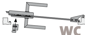
WC-Zylinder Für nach außen öffnende Tür Einsetzbar in Schlosskasten PZ WC-Zylinder an Schlossgegensseite 99035
