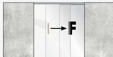
1 Tür links, nach rechts öffnend, 1 Element rechts, Breite bis 2310 mm
