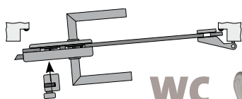
WC-Zylinder Für nach innen öffnende Tür Einsetzbar in Schlosskasten PZ WC-Zylinder an Schlossseite 99034
