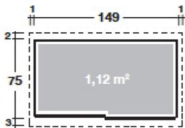
Grundriss Gartenschrank 157
