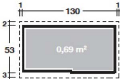
Grundriss Gartenschrank 135
