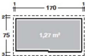
Grundriss Gartenschrank 177
