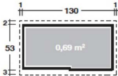
Grundriss Gartenschrank 135
